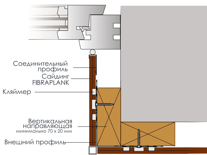
Внешний асимметричный угловой профиль
